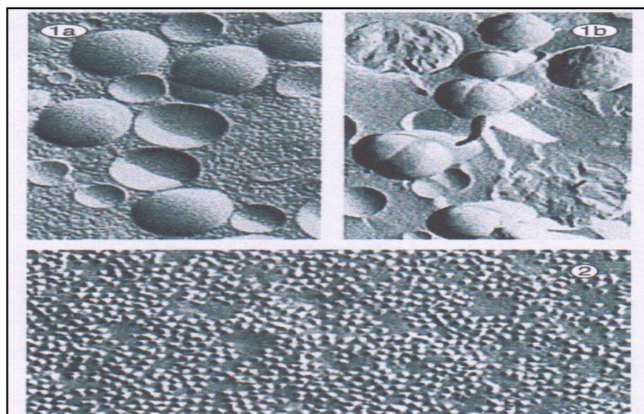
Figure 8. Clichés obtenus par cryofracture.
