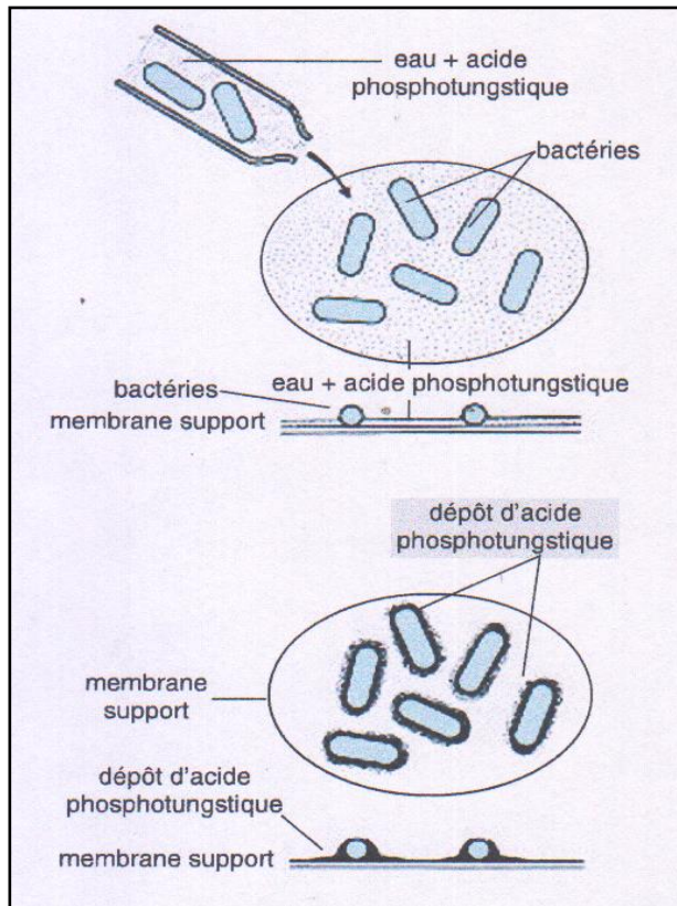
Figure 5. Principe de la coloration négative
