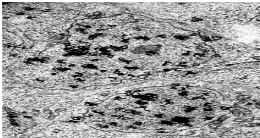
Figure 10. Cliché d'autoradiographie en microscopie électronique
